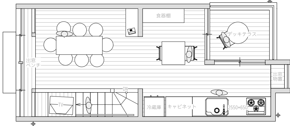
2階平面図
