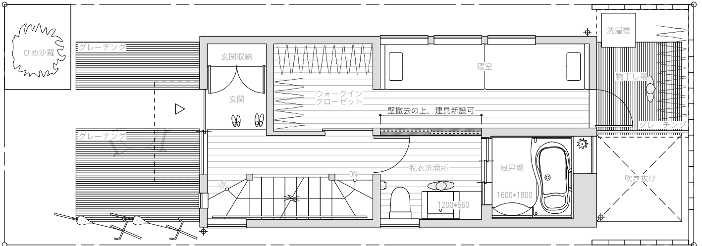
1階平面図
